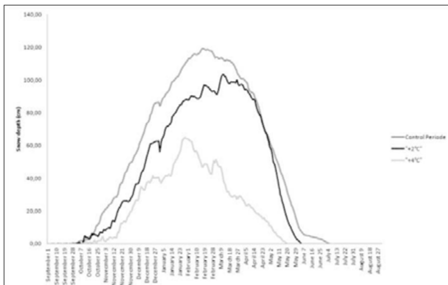
Figura 2. Evolución del espesor de nieve a 2.500 m de altitud en función de diferentes escenarios de cambio climático (periodo control, +2°C y +4°C) en función del calendario invernal.
